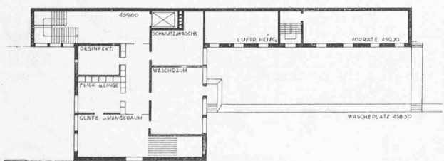
Erdgeschoss mit Eingängen. — 1 : 600.
