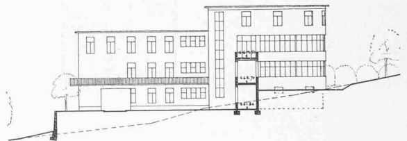
Nordwestansicht, darüber Erdgeschoss und 1. Stock, 1 : 700.
