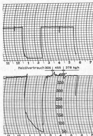
Abb. 6. Druck- und Temperaturverlauf bei einem Versuch mit dem Sulzer-Einrohr-Hochdruck-Dampferzeuger. Oben: Druckverlauf bis 90 at (von 12.55 bis 14.30 h Dampferzeuger abgestellt). Unten: Temperaturverlauf.
