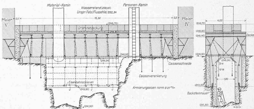
Abb. 42. Unterfahrung einer Caissonschnide mit Eisenbeton am Stauwehr Augst-Wyhlen. — 1 : 200. Entwurf und Ausführung A. G. Conrad Zschokke, Genf. [Aus der „S. B. Z.“ vom 12. April 1913.]
