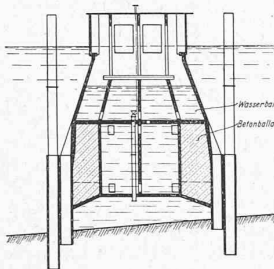
Abb. 45. Querschnitt 1 : 800. Pfeilergründung der Eisenbahnbrücke über den Kleinen Belt, Dänemark. Patent Grün & Biflinger. [„S. B. Z.“ 26. Dez. 1931.]
