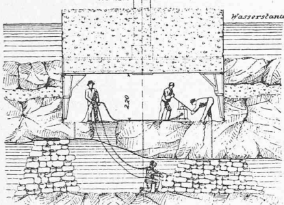
Abb. 41. Unterfahrung einer Caissonschnide durch Taucher. Brücke über die Dordogne. [Aus der „S. B. Z.“ vom 25. August 1883.]
