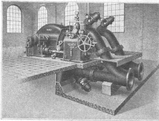
Eine der Pelton-Turbinen des Sernt-Niederbachwerkes. 4 Düsen. — 7400 PS unter 215 m Gefälle. — 500 t/min.
