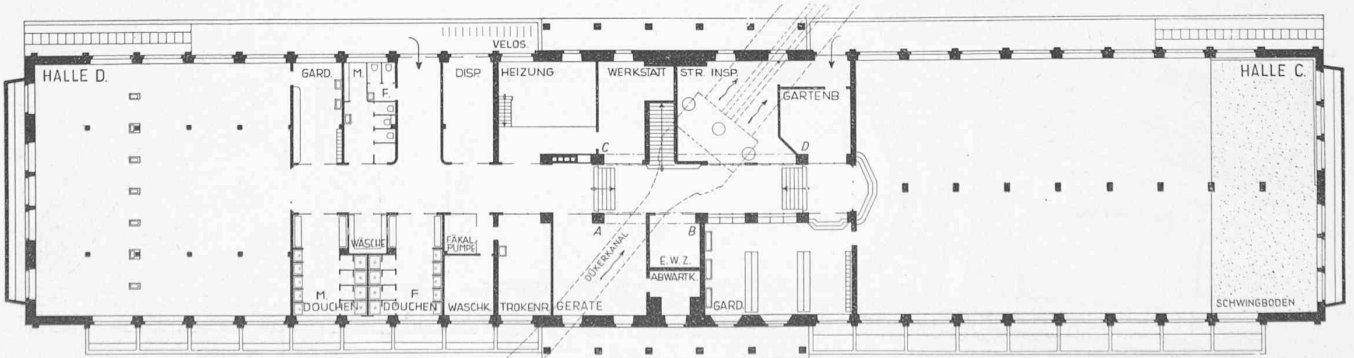
Abb. 5 bis 7. Grundriss vom Untergeschoss, darüber Querschnitte (samt S. B. B.-Tunnel und Düker). — Masstab 1:500.
