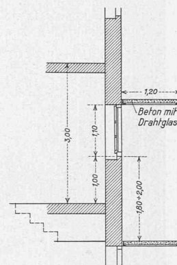
Abb. 2 (rechts). Vertikalschnitt durch Wand und Aussengänge. Massstab 1:100.
