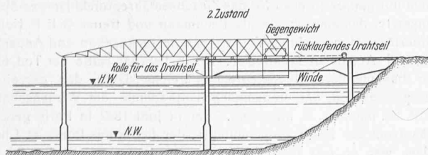
Verschiebbare eiserne Rüstung zum Bau von Eisenbetonbrücken in Marokko.
