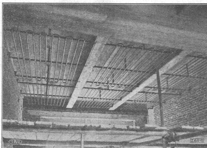
Eine Deckenheizung in Montage. — Die Heizschlangen liegen noch offen.
