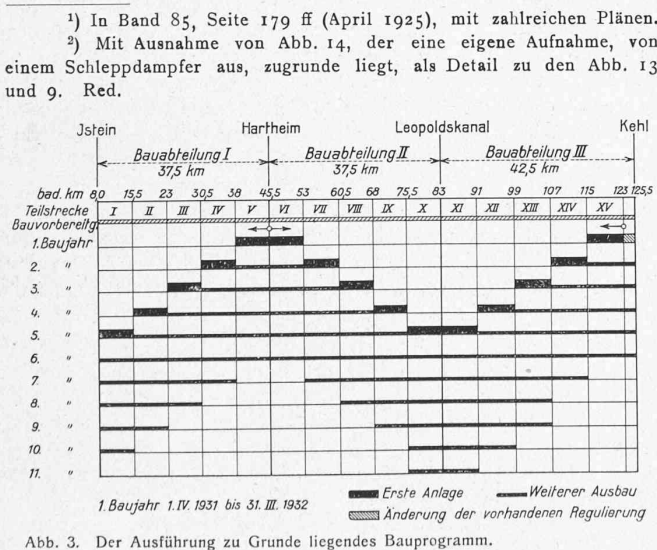
Abb. 3. Der Ausführung zu Grunde liegendes Bauprogramm.
