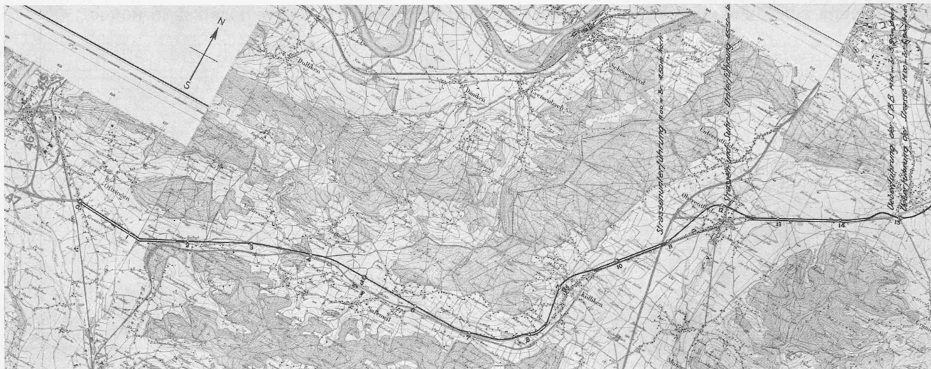
Abb. 27. Fernverkehrstrasse Bern-Zürich, Teilstrecke Kreuzstrasse-Innlauf (Km. 0 bis 15). Ing. Rob. Naef, Zürich. — Masstab 1 : 80 000.
