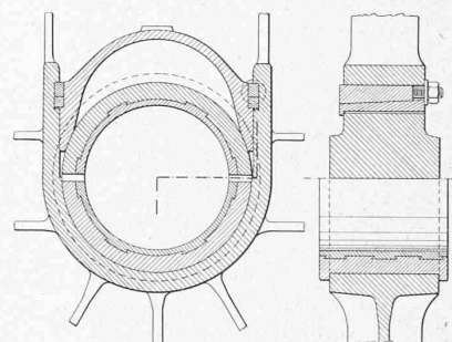
Abb. 8. Lagerdeckel-Befestigung für schnelllaufende, doppeltwirkende Sulzer-Dieselmotoren.
