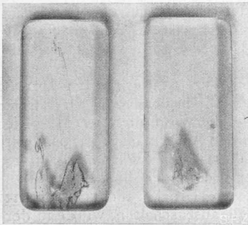
Abb. 13. Kavitations-Korrosionen an Glas.
