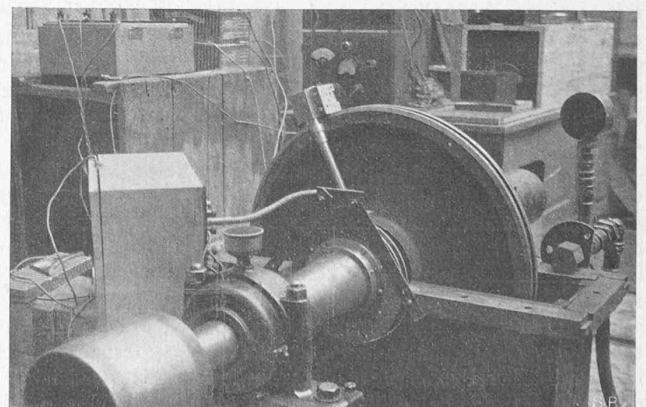
Abb. 23. Die Piezoquarz-Zelle an der Scheibe für Tropfenschlagversuche.
