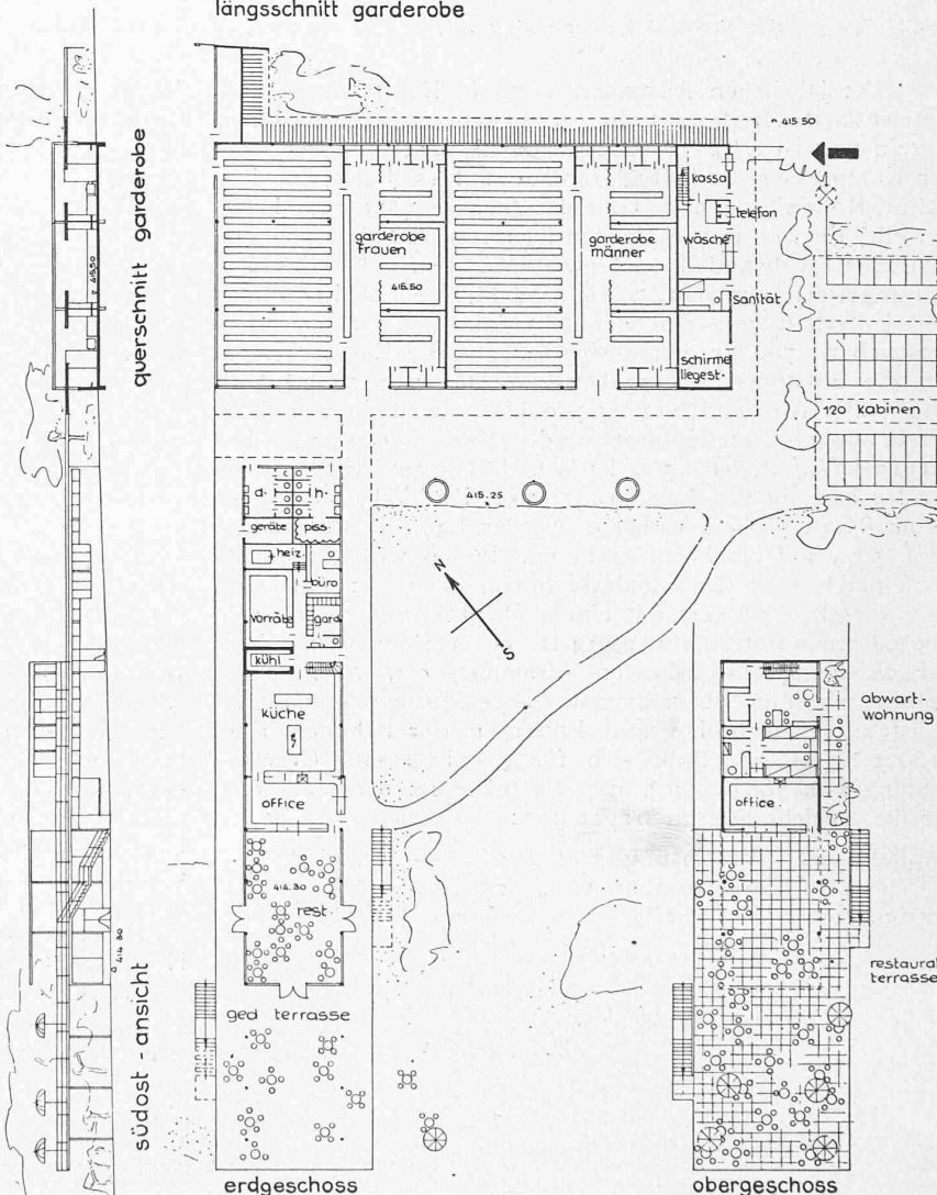
längsschnitt garderobe
