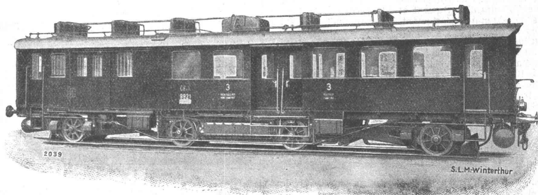
300 PS Diesellokomotive im Betrieb auf der Strecke Glarus-Uznach der S. B. B., ausgerüstet mit Geschwindigkeitswechselgetrieben System „S. L. M.-Winterthur“.
