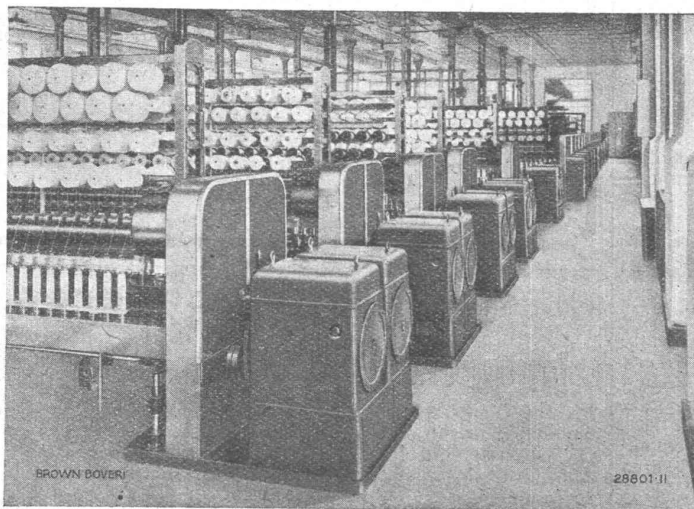
Antrieb von doppelten Baumwoll-Ringspinnmaschinen mit Dreiphasen-Komm-tatormotoren.
