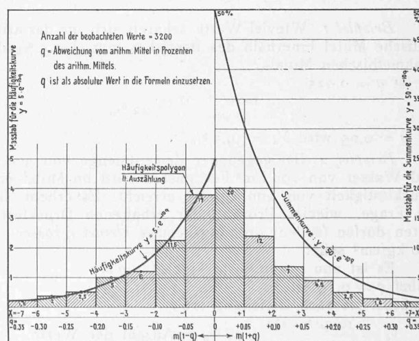
Abb. 7. Häufigkeitspolygon, Häufigkeitskurve, Summenkurve.
