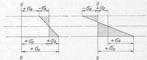
Abb. 7. Spannungsverlauf, links mit \sigma_b < \sigma_z , rechts \sigma_b > \sigma_z .
