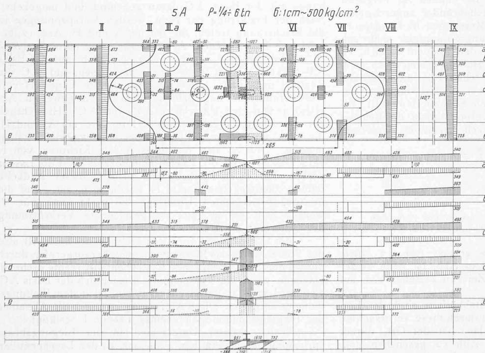
Abb. 4 (oben) und 5 (unten). Gruppen 3 (3A, Lasche mit Stufen, ohne Kehlnähte) und 5 (5A, gezackte L., ohne Kehlnähte).
