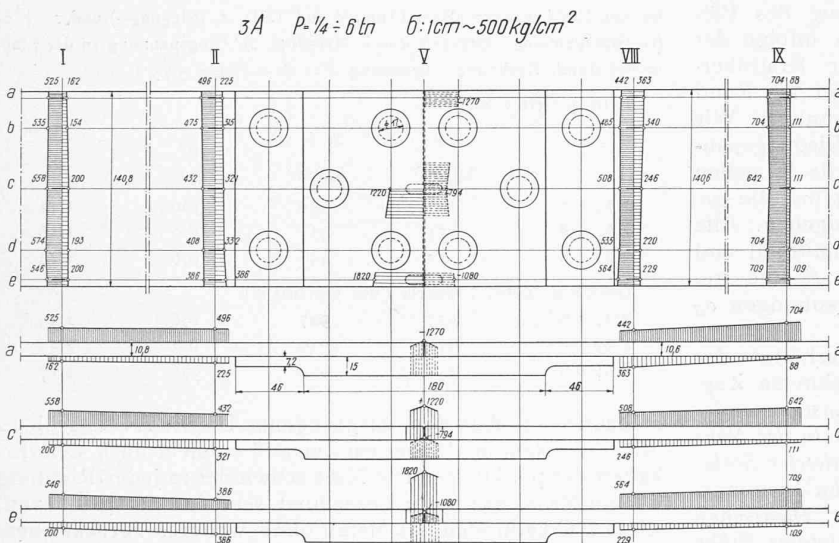
Abb. 7. Spannungsverlauf, links mit \sigma_b < \sigma_z , rechts \sigma_b > \sigma_z .
