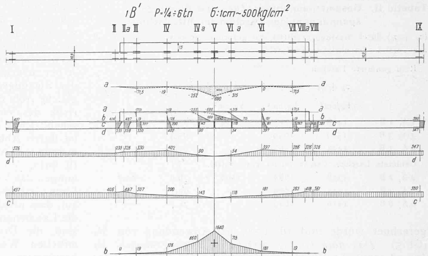
Abb. 10 Stab 1 B, Gruppe I. — Messungen im Längsprofil. Lasche ohne Kehlkräfte.
