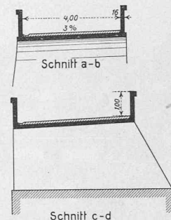
Schnitt a-b
