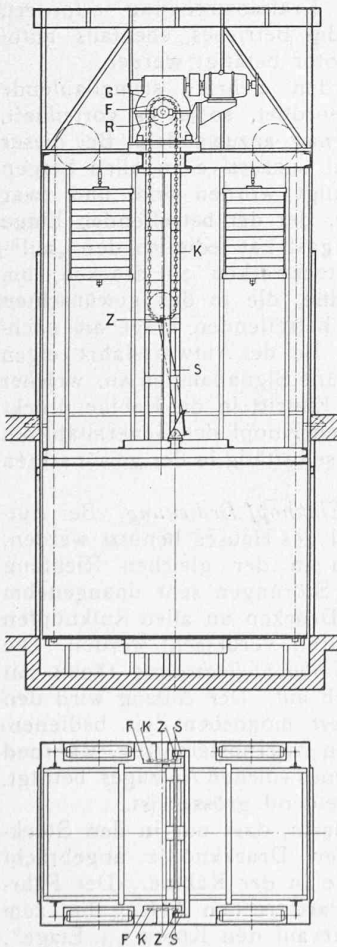
Abb. 10. Antriebsmaschine oben.
