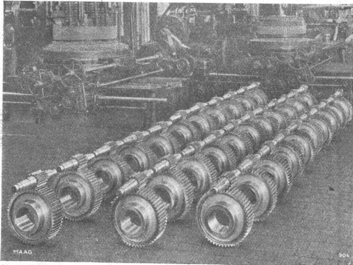
Tramgetriebe mit gehärteter und geschliffener Verzahnung für die Strassenbahn der Stadt Zürich.
