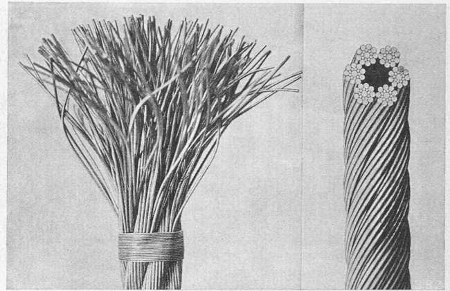
Abb. 18. Gewöhl. Stahldrahtseil, nicht vorgeformt. Abb. 19. Vorgeformtes Seil.
