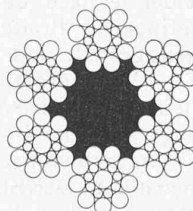
Abb. 22. Seale-Seil.
