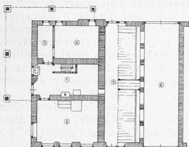
Abb. 15. Erdgeschoss.
