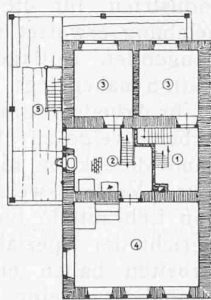
Abb. 16. Erster Stock.
