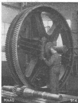
Maag-Pfeilradgetriebe für Förderanlage, Charbonnages Elisabeth, Auvérais Belgien. (Ritzelverzahnung, gehärtet und geschliffen.)
