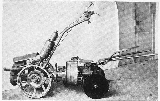
Abb. 4. Bodenfräse System „Simar“ (Genf), kombiniert mit Seilwinde für Pflügen und Reberg-Bearbeitung.
