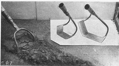
Abb. 1. Ziehhackgeräte System Wolf für Arbeit im Rückwärtsgang.
