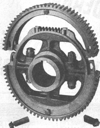
Abgefedertes Maag-Traktionsrad, Type Protex (Montreux-Oberlandbahn)
