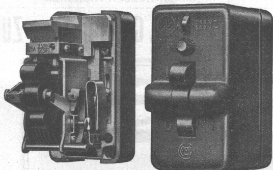
Installations-Selbstschalter 500 Volt, 25 Amp. mit Nulleiterklemme
