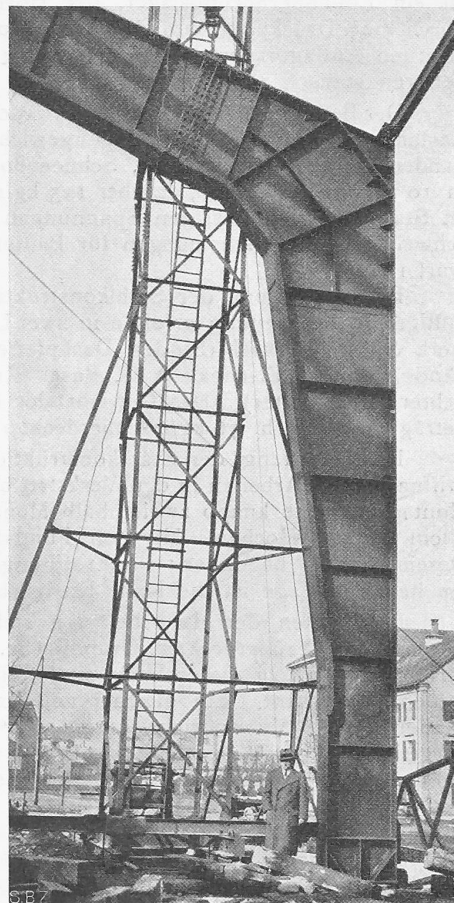
Abb. 3. Montage eines Binders.
