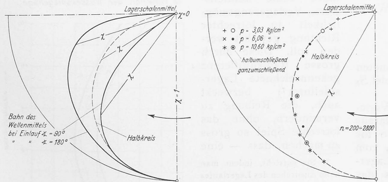
Abb. 1. Theoretische Bahn des Wellenmittels nach Stieber. Gestrichelt: Halbkreis.
