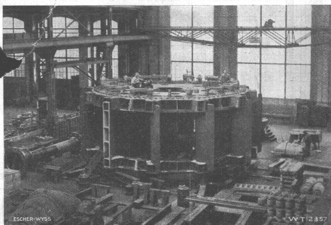
AAREKRAFTWERK KLINGNAU
