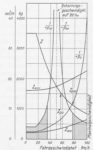
Abb. 1. Charakterist. Kurven für einen 410 PS Diesel-elektr. Triebwagenzug v. 70 t. Z = Zugkraft am Radumfang, Zwo = Fahrwiderstand auf der Ebene, Zw20 = Fahrwiderstand auf 20 % Steigung mit 12 km/h Gegenwind. Zp = Beschleunigungs- bez. Verzögerungskraft. +p = Beschleunigung, -p = Verzögerung.
