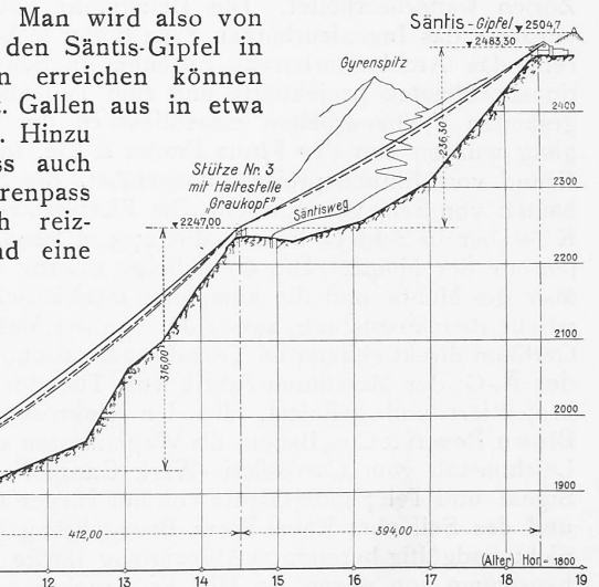
Abb. 2. Längenprofil 1 : 10 000 (nicht überhöht).
