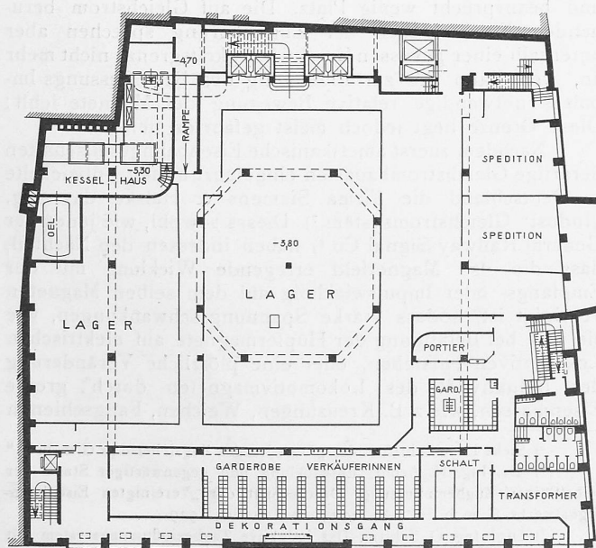
Abb. 1. Kellergeschoss. — Masstab 1 : 600.
