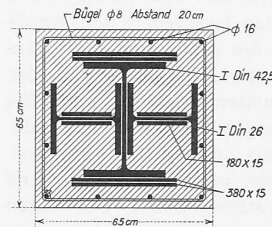
Abb. 16. Stützen-Querschnitt. Masstab 1:25.
