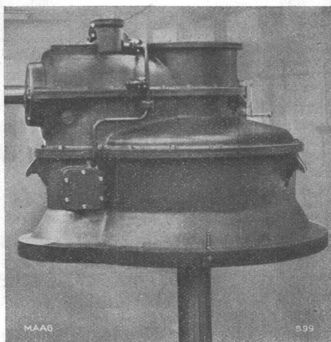
Maag-Drehzahl-Erhöhungsgetriebe (Stirn-Kegelradgetriebe) zwischen Wasserturbine und Drehstromgenerator zur Uebertragung von 560 PS bei 144/750 Uml./min.
