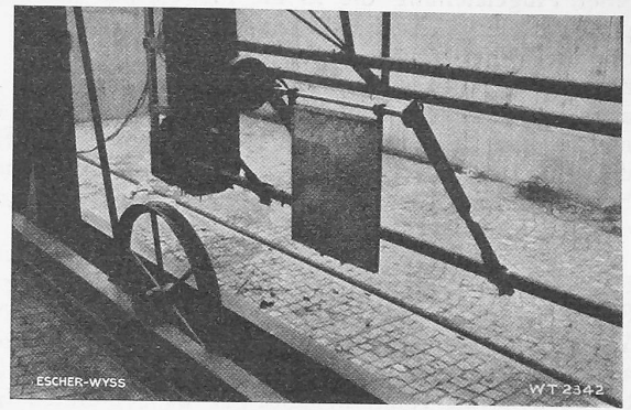
Abb. 5. Fahne mit Pendel zur Bestimmung der Strömungsrichtung; Befestigung an der Flügelstange.
