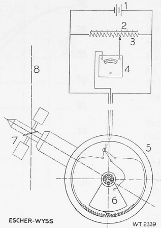
Abb. 6. Schema der elektrischen Winkelübertragung. — Legende: 1 Batterie, 2 Eichskala, 3 Vergleichswiderstand, 4 Millivoltmeter, 5 Pendelkörper auf der Flügelstange, 6 Pendel mit Kontaktfeder, 7 Flügel, 8 Messebene.
