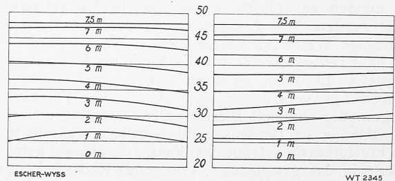
Abb. 7. Verteilung der gemessenen Strömungswinkel über die beiden Einlauföffnungen, für verschiedene Höhenlagen.
