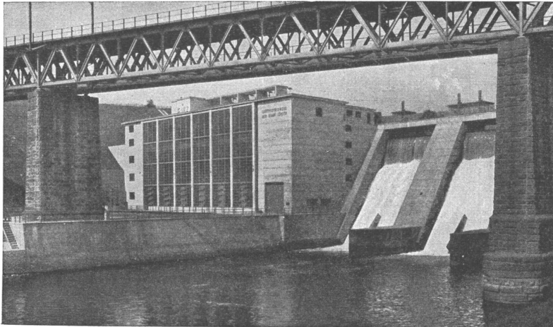
Kraftwerk Wetzlingen der Stadt Zürich Bedachung des Maschinenhauses ca. 1200 m 2 .
