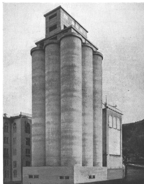
Getreide-Silo Steiners Söhne Malters Inhalt 3300 Tonnen
