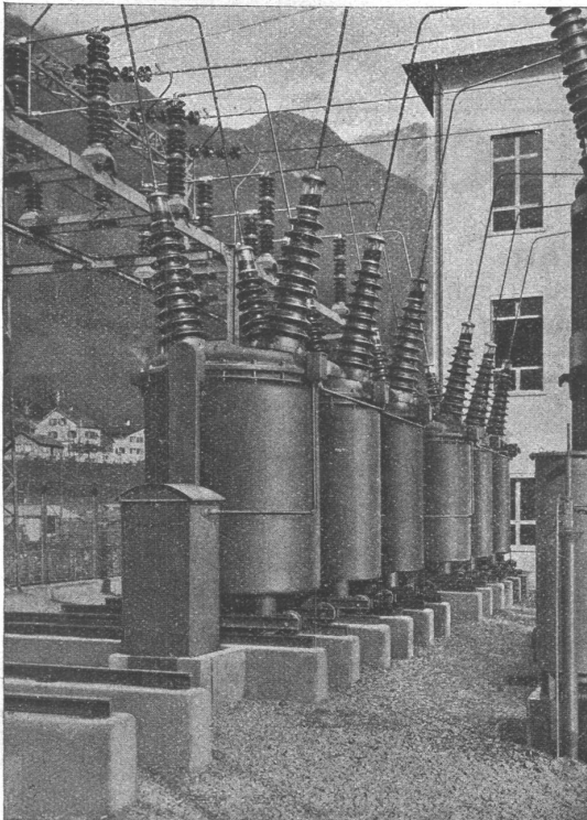
150 kV Oelschaltergruppen
