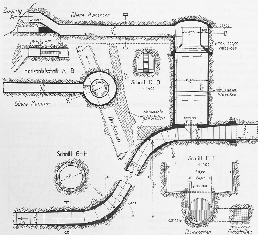
Abb. 18. Uebergang des Stollens in den Druckschacht mit Wasserschlössli und oberer Kammer. — 1 : 800.
