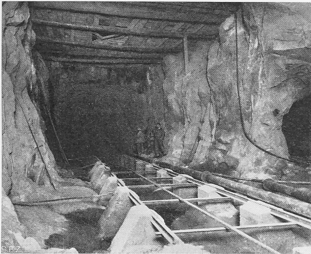
Abb. 17. Abzweigstelle des Druckschachtes (links) vom Richtstollen (rechts); über dem Gerüstboden der Wasserschlössli-Steigschacht.
