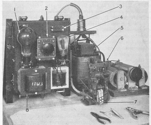
Abb. 3. Thyatron-Apparatur für Punktschweißung (1 kVA), Deckel abgehoben. 1 Thyatron, 2 Gitterspannungsregler, 3 Kondensatoren, 4 Gleichrichter, 5 Schweißtransformator, 6 Schweißser, 7 Kontrollkontakte, 8 Hilfstransformator.
