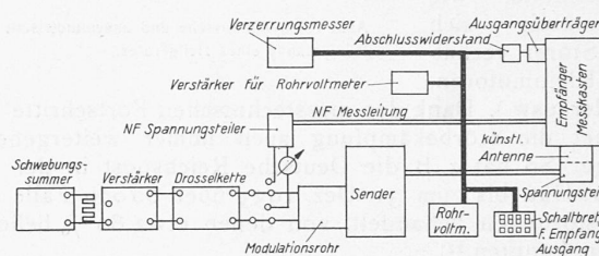
Abb. 4. Schema einer Rundfunkempfangs-Messeinrichtung.
