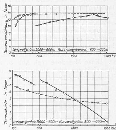
Abb. 5 und 6. Gesamtverstärkung und Trennschärfe.
