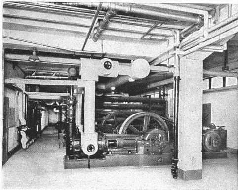
Abb. 18 (links). Kompressorenraum.
