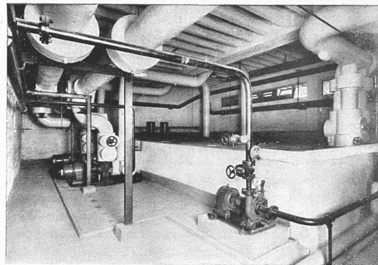
Abb. 19 (rechts). Kältespeicher.
