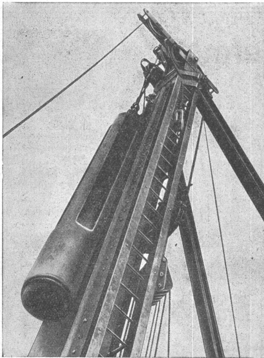
Franki-Ramme mit 3000 kg Bär
