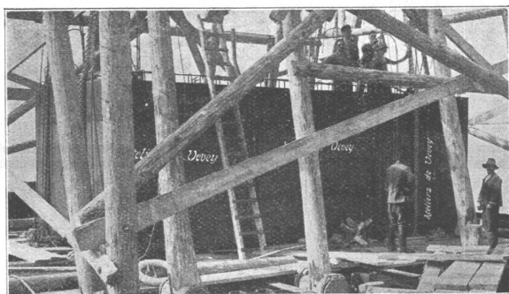
Druckluftcaisson für den neuen Hafen von Vevey.
