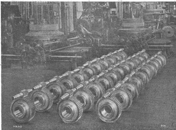
Teillieferung von Tramgetrieben mit gehärteter und geschliffener Verzahnung für die Strassenbahn Zürich.
