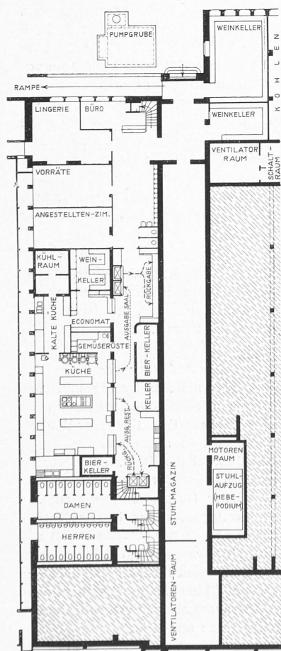
Abb. 5. Küchen-Untergeschoss (Nordflügel).
