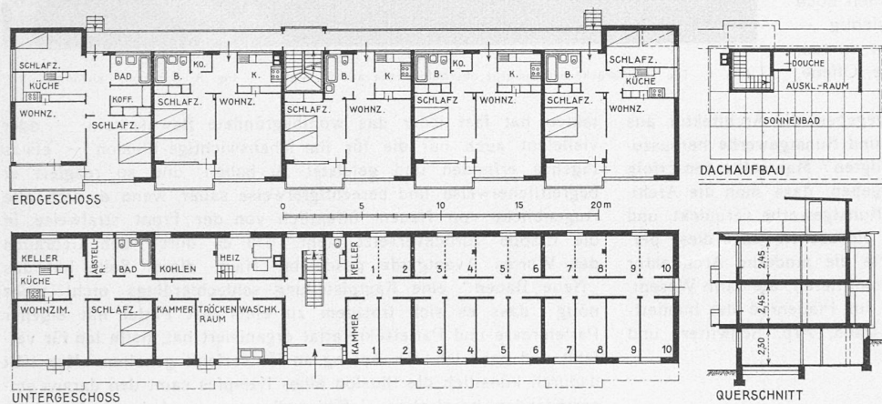
Abb. 1. Grundrisse und Schnitt. — Masstab 1:400.
