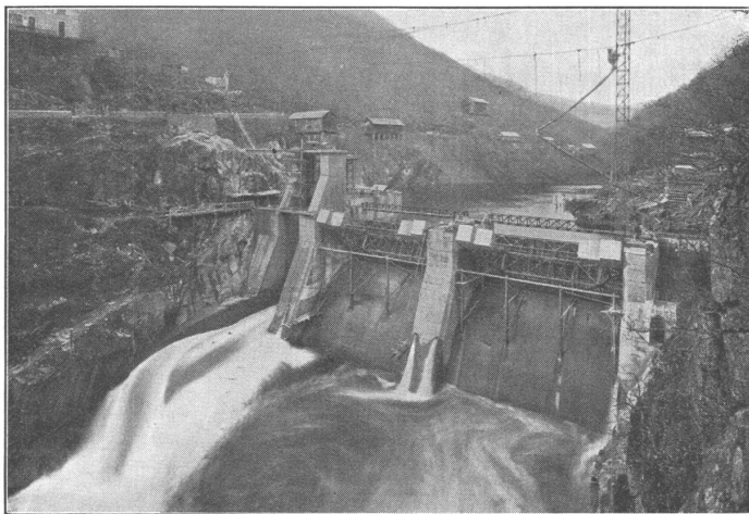
Wehranlage La Cadène an der Truyère, zwei automatische Segmentschützen je 18 \times 6 m.
