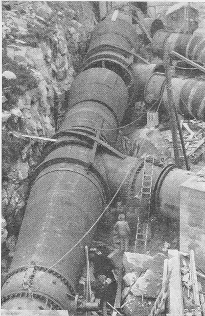
Abb. 29. Verteilung mit Abzweigungs-Verstärkungen (im Bau).
