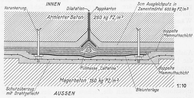
Abb. 37. Einzelheiten der Abdichtung des Maschinenhauses.
