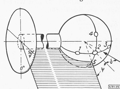
Abb. 2. Staukugel (schraffiert die Bezugsebene).
